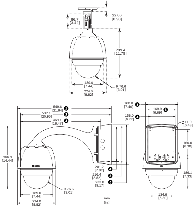
Şek. 2: AUTODOME 7000 serisi Boru, Askı montajları
